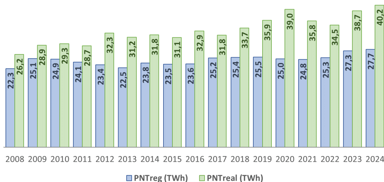
Figura 11 – Perdas Não Técnicas Reais e Regulatória sobre BT Faturado - TWh (2024)
