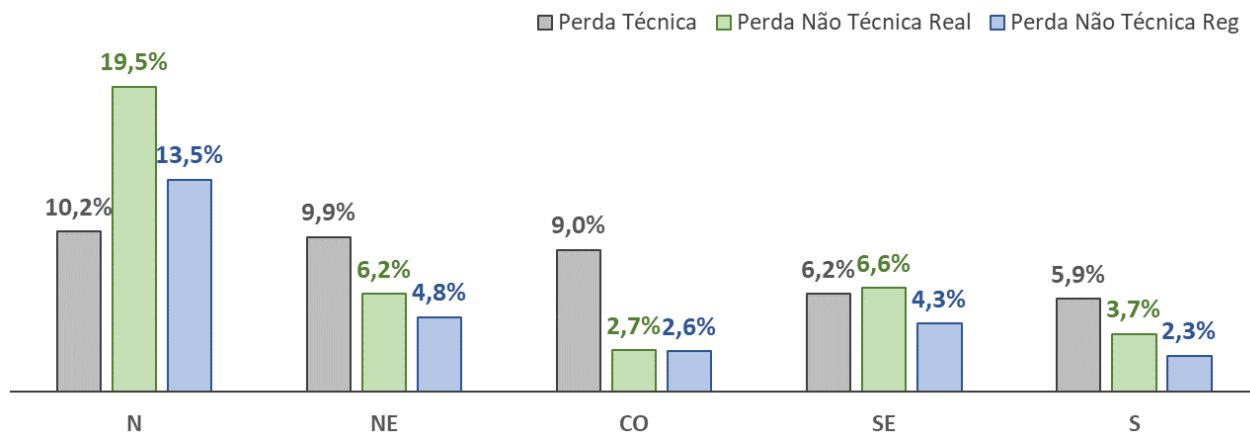
Figura 5 – Perdas Técnicas Regulatórias, Não Técnicas Reais e Regulatórias sobre a Energia Injetada (2024)
