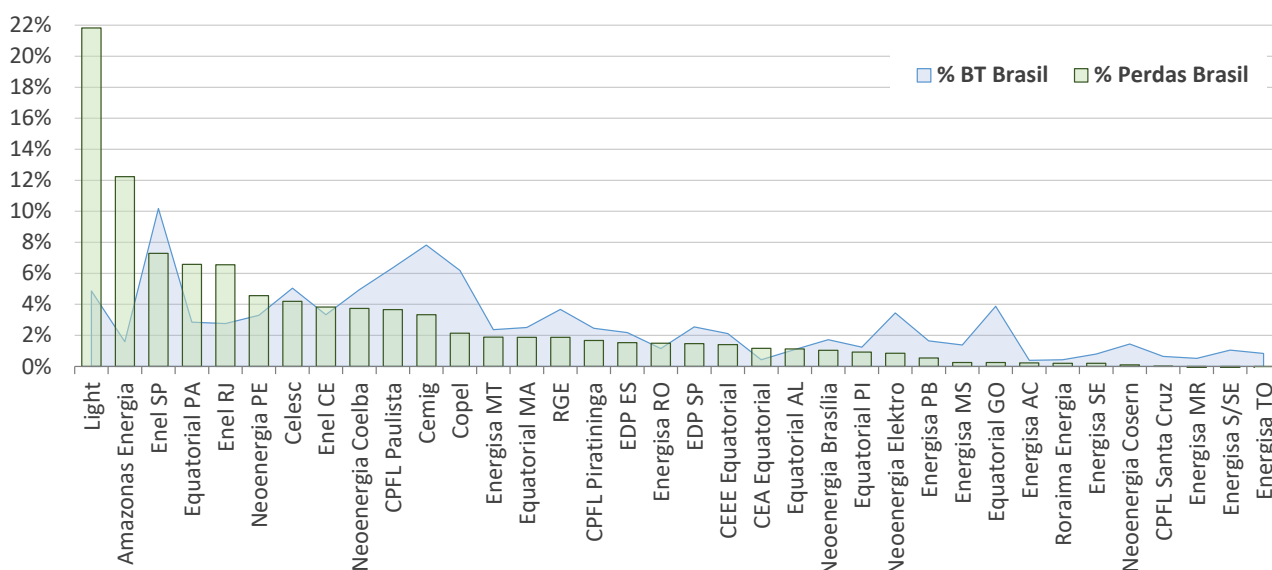
Figura 9 – Participação das Perdas Não Técnicas Reais e do Mercado BT (2024)
