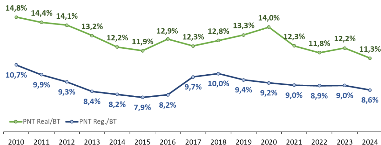
Figura 12 – Perdas Não Técnicas Reais e Regulatórias sobre BT Faturado (média simples)
