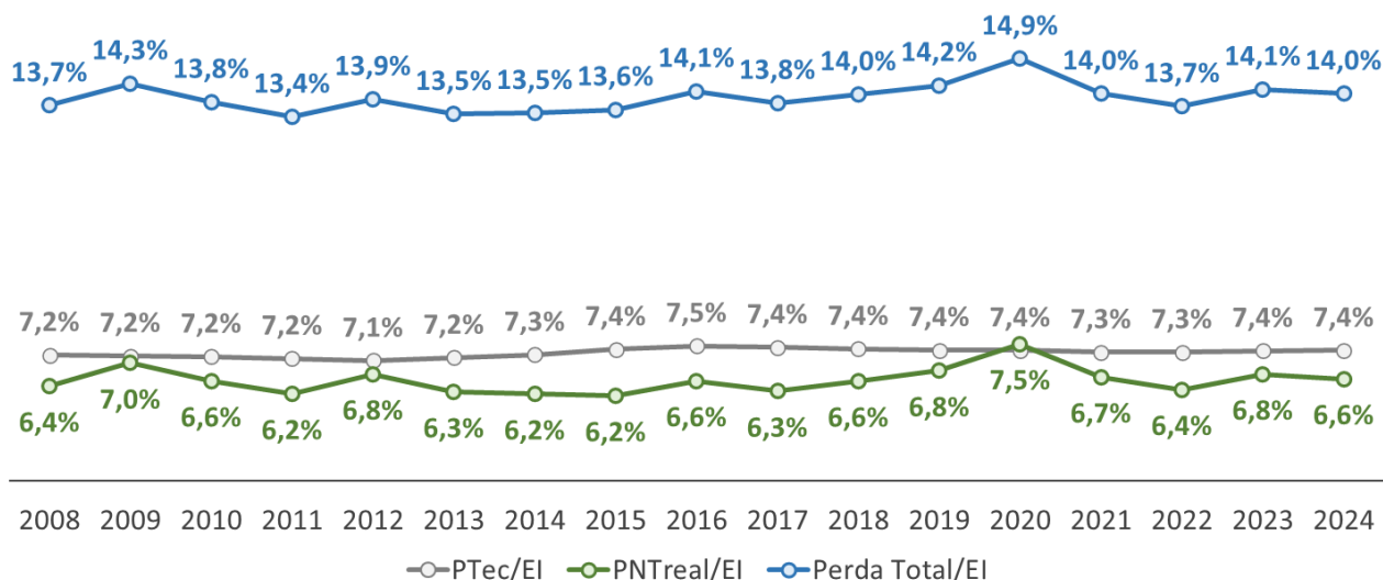
Figura 3 – Perdas sobre a Energia Injetada (2008-2024)
