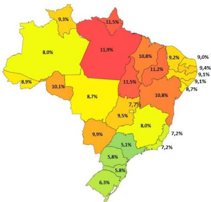
Figura 6 – Perdas Técnicas Regulatórias sobre Energia Injetada (2024)
